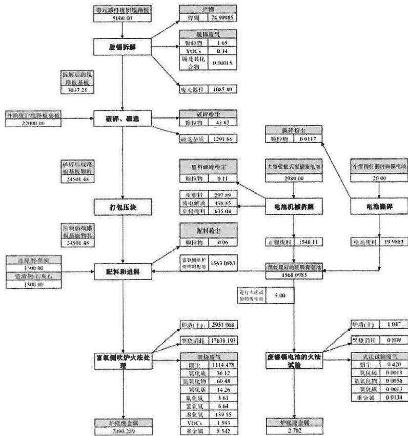
项目废弃镉镍电池工艺处置工艺流程图
